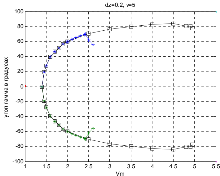
Рис.1. Положення стійких коливань.
