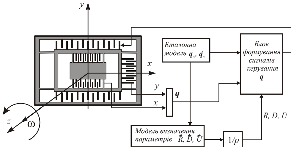
Рис. 1 Система адаптивного керування первинними коливаннями чутливого елемента мікромеханічного гіроскопа
