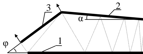
Рис.1. Оптическая схема трёхзеркального резонатора лазера и ход луча в нём: 1 и 2 – высокоотражающие зеркала, 3 – выходное зеркало
