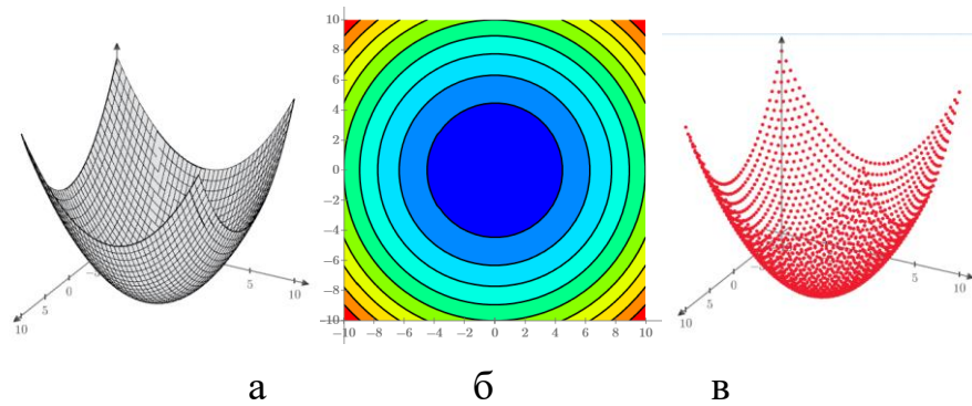
Рис. 3.59. Типи тримірних графіків: а – поверхні; б – контурний; в – точковий
