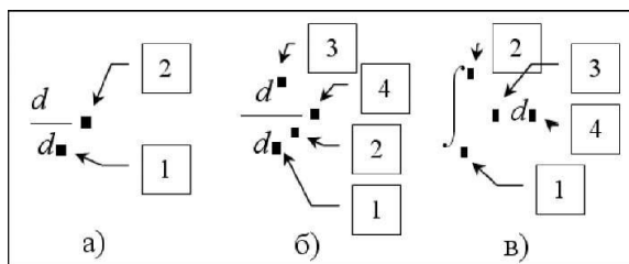
Рис. 3.13. Шаблиони операторів диференціювання та інтегрування
