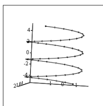
Рис. 3.54. Графік просторової спіралі
