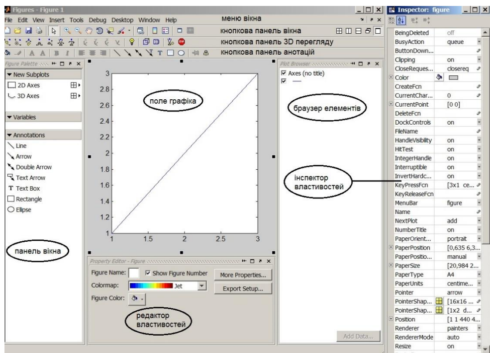
Рис. 4.11. Графічне вікно
