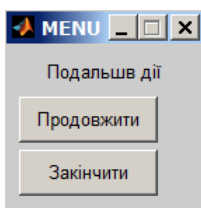
Рис. 4.8. Меню завдання 4.2.6
