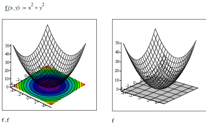
Рис. 3.58. Зображення поверхні з «тінню».
