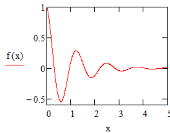
Рис. 3.33. Відкоригований графік
