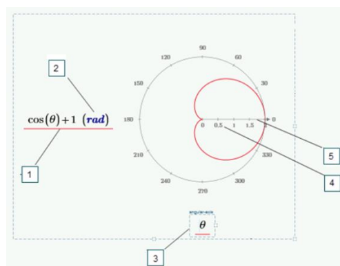
Рис. 3.41. Шаблон графіка в полярних координатах
