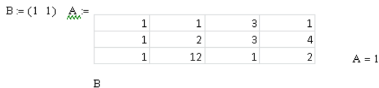
Рис. 3.83. Компонент Excel
