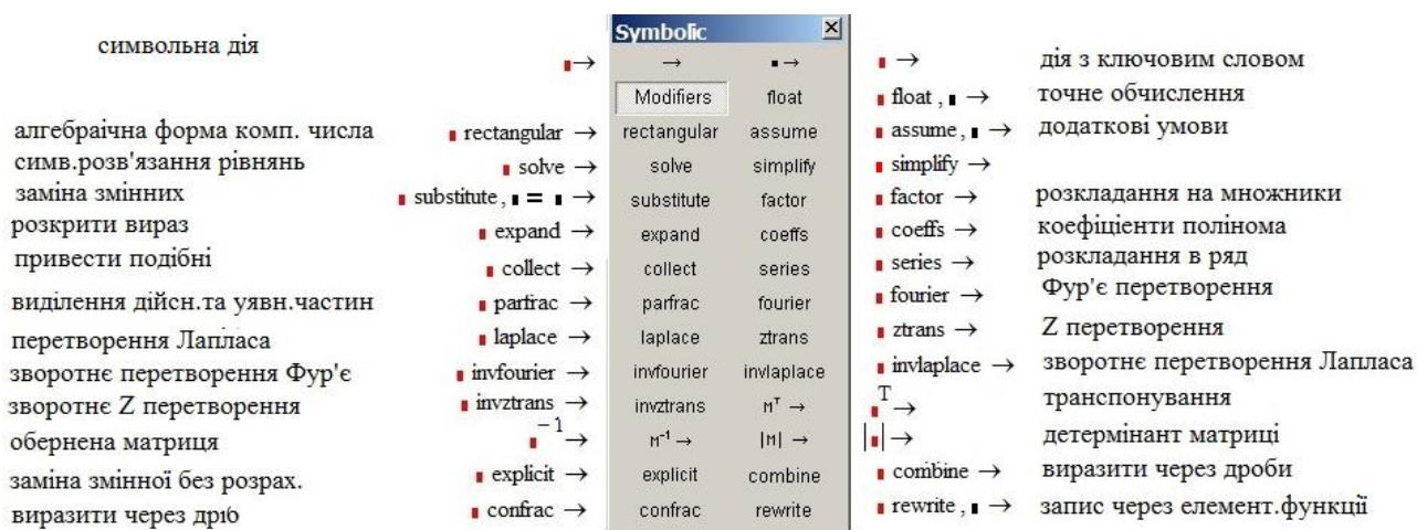
Рис. 3.72. Панель символьних перетворень
