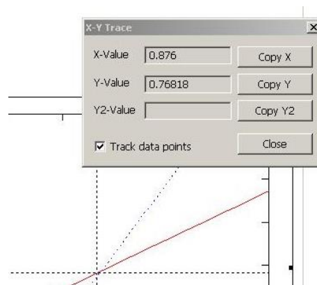
Рис. 3.44. Режим Trace
