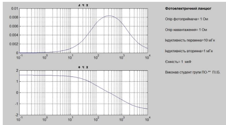
Рис. 4.15. Вигляд вікна завдання 4.3.8
