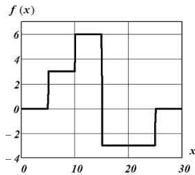
Рис. 3.27. Функція до завдання 3.1.9 Рис. 3.28. Область до завдання 3.1.10
