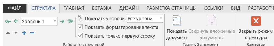
Рис. 1.14. Стрічка структури
