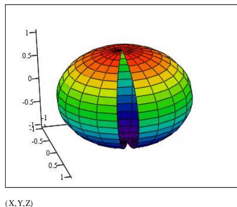
Рис. 3.67. Сфера завдання 3.4.2
