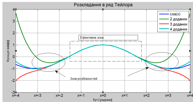
Рис. 4.16. Зображення завдання 4.3.9
