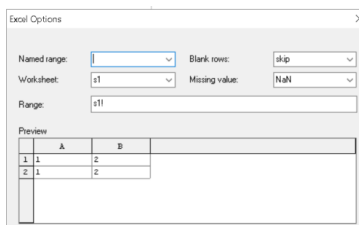
Рис. 3.81. Діалог файлів MS Excel : а – вікно діапазону; б – позначка в документі
