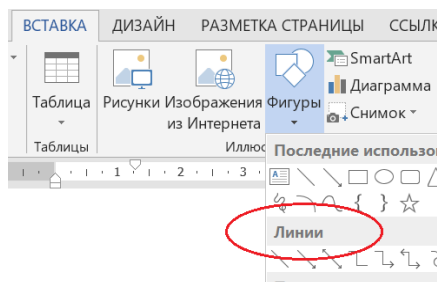
Рис. 1.4. Фігури
