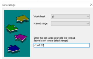
Рис. 3.78. Імпорт з MS Excel : а – вікно визначення діапазону; б – позначка в документі
