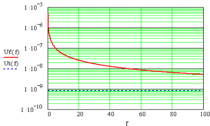
Рис. 3.45. Графік прикладу 3.3.2
