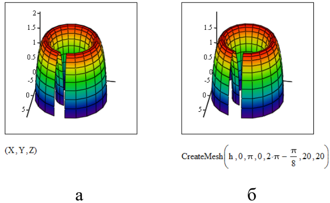
Рис.3.66 Зображення торичної поверхні: а – параметричне; б – функцією CreateMesh
