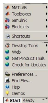
Рис. 4.2. Кнопка Start
