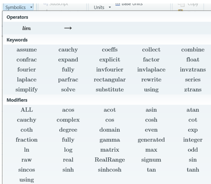
Рис. 3.75. Панель символічних перетворень
