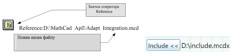
Рис. 3.29. Шаблон імпортування
