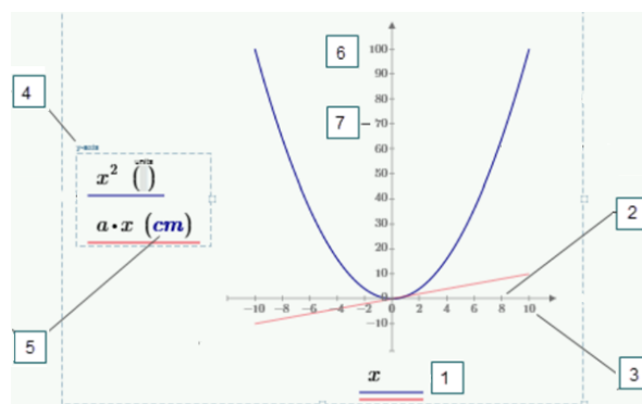
Рис. 3.39. Поле графіка в декартових координатах з маркерами:
