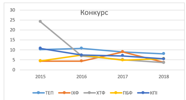
Рис. 1.11. Завдання 1.2.2
