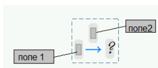
Рис. 3.76. Універсальний шаблон
