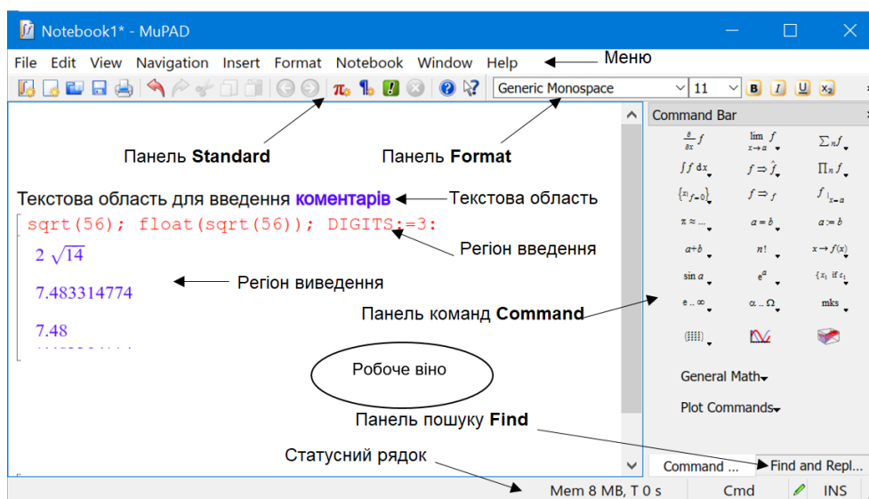
Рис. 4.19. Оболонка MuPAD
