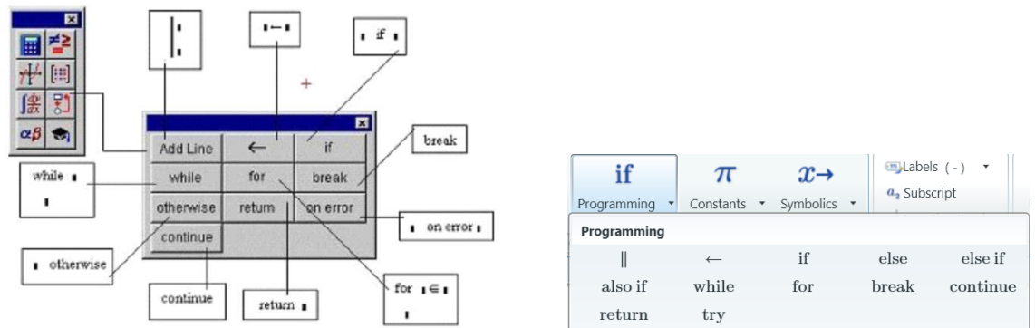
Рис. 3.27. Панель програмування
