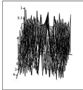
Рис. 3.63. Первинне зображення
