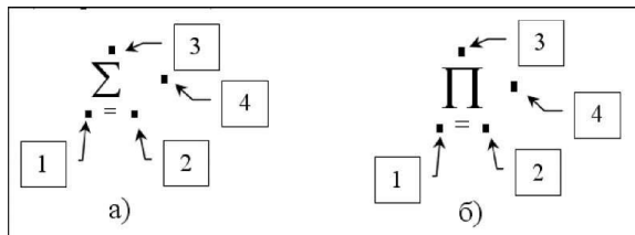
Рис. 3.11. Шаблони операторів сум та доданків: а – шаблон сум; б – шаблон доданку [1]
